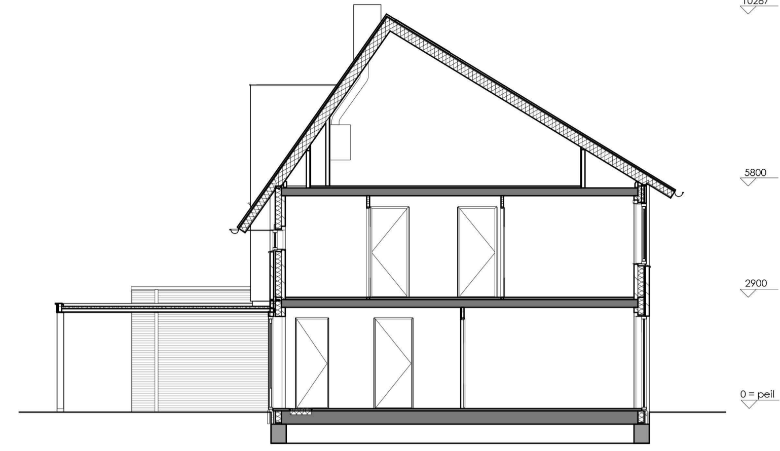
Doorsnede A-A
