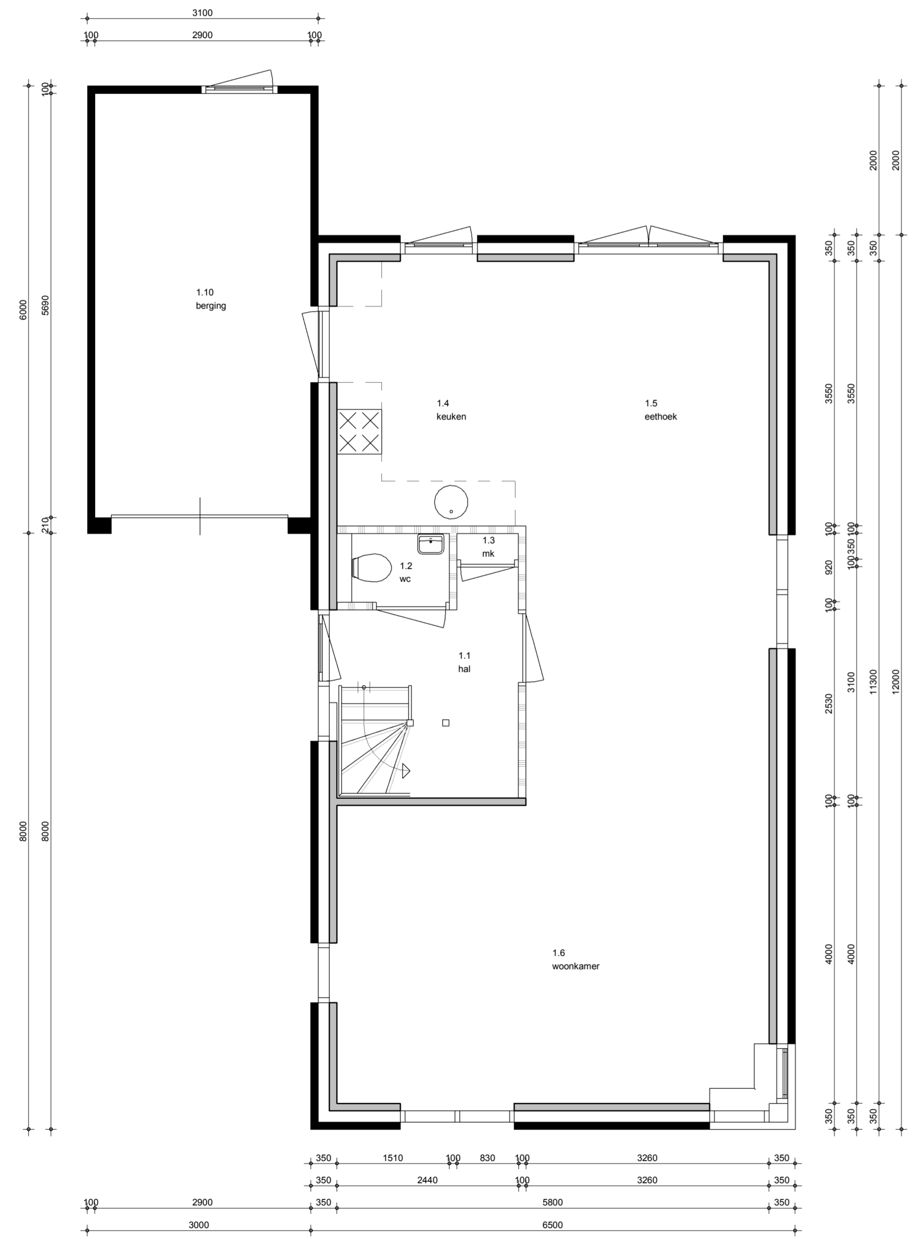
begane grond
