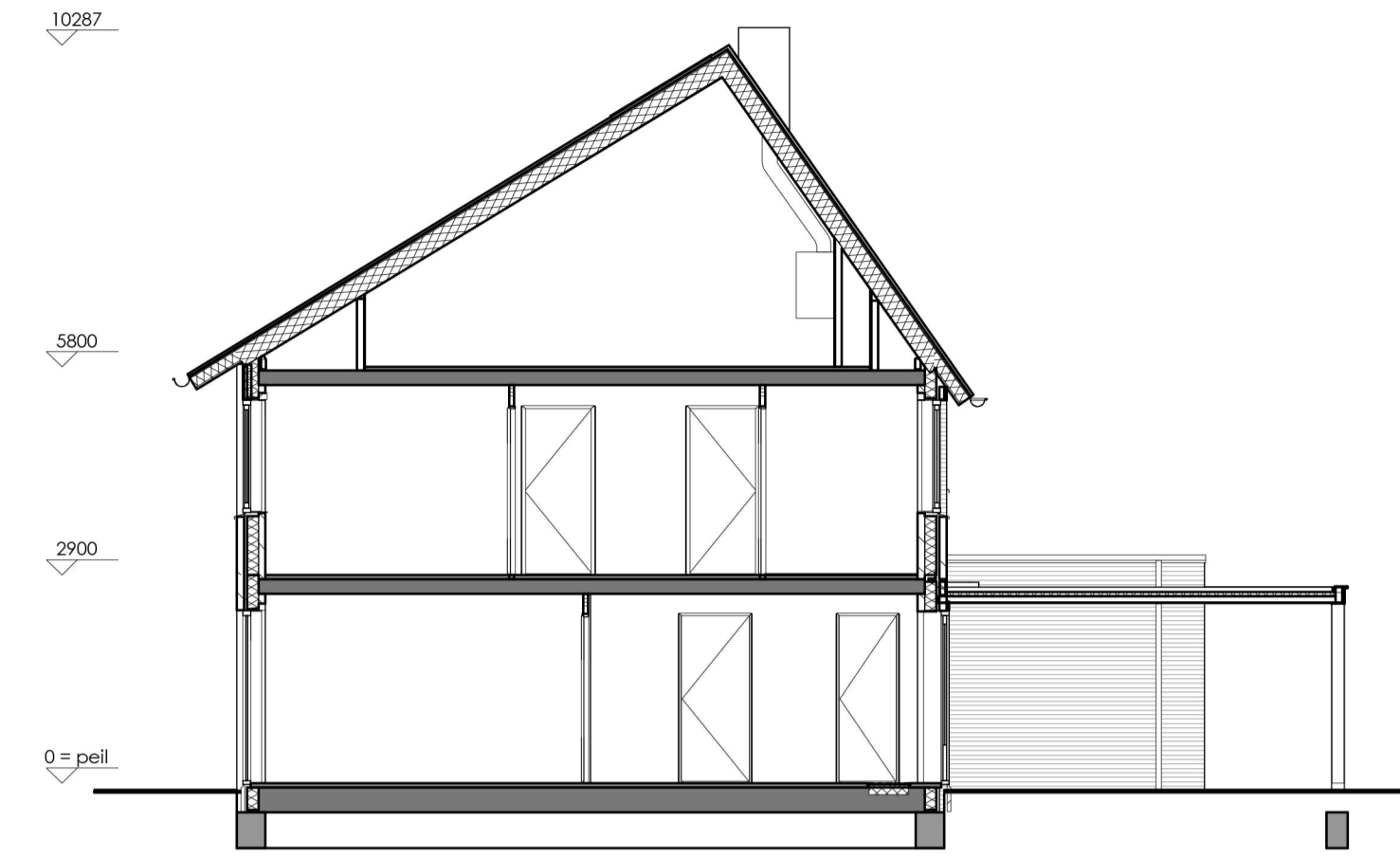
Doorsnede A-A
