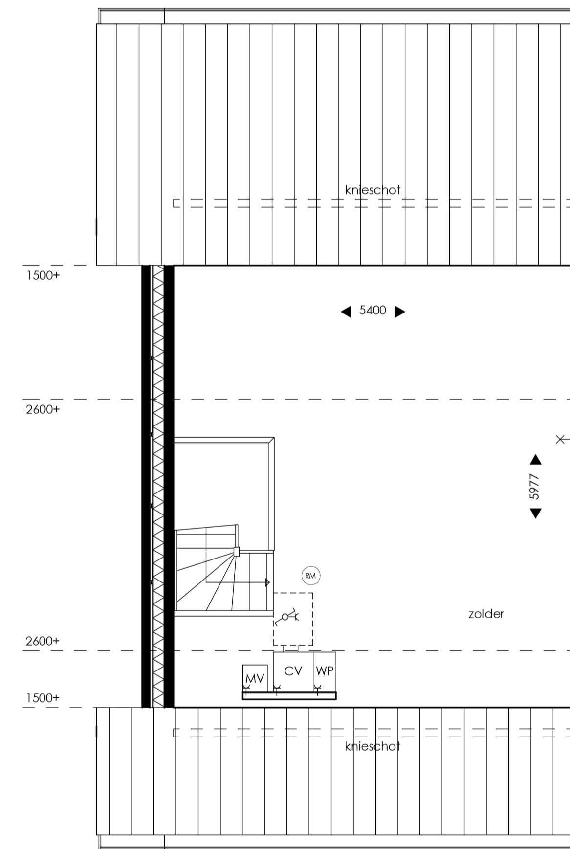
Tweede verdieping
