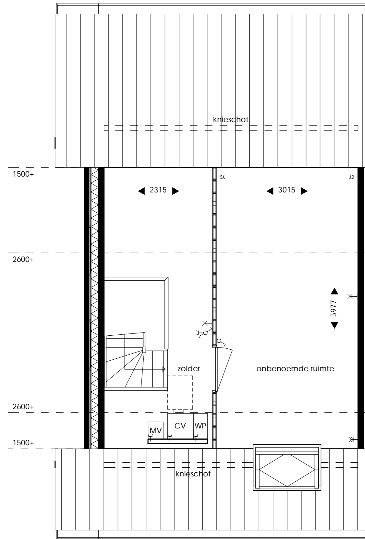
Tweede verdieping
